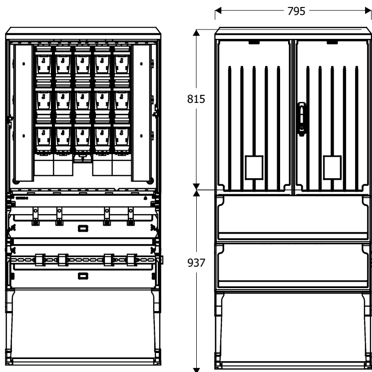
Widok złącza
