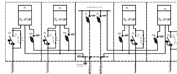
Schemat elektryczny
