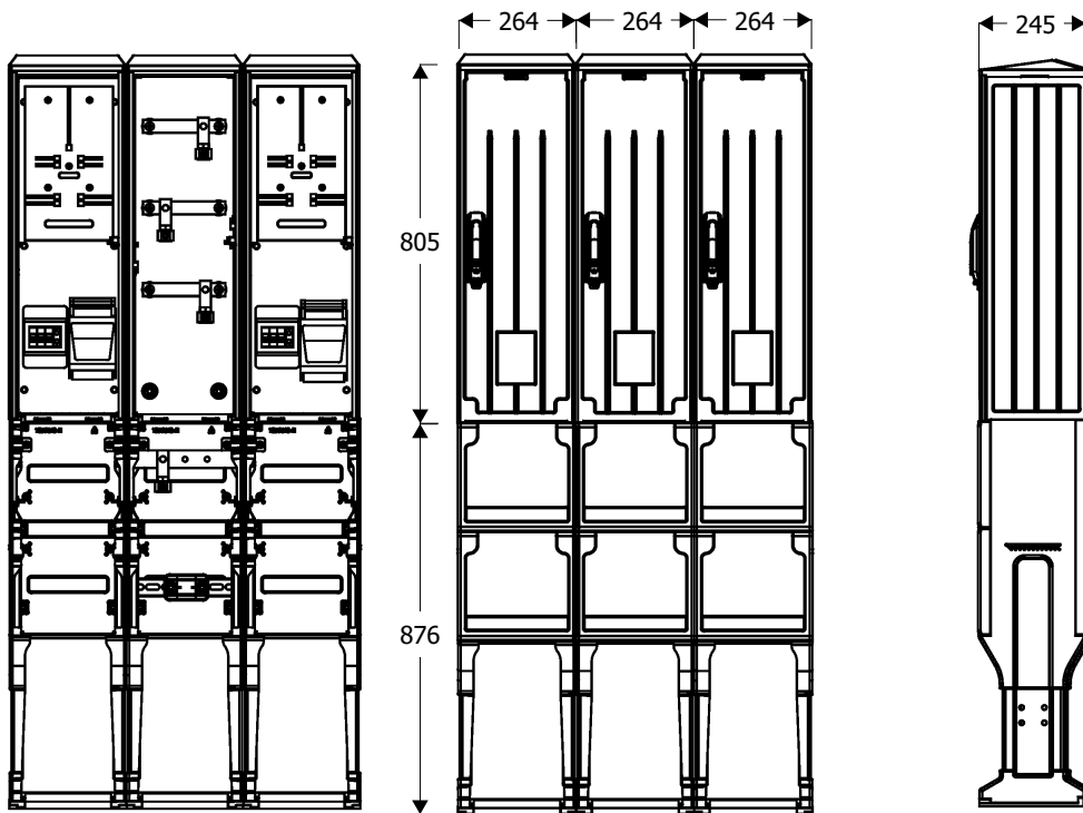
Widok złącza
