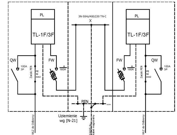
Schemat elektryczny
