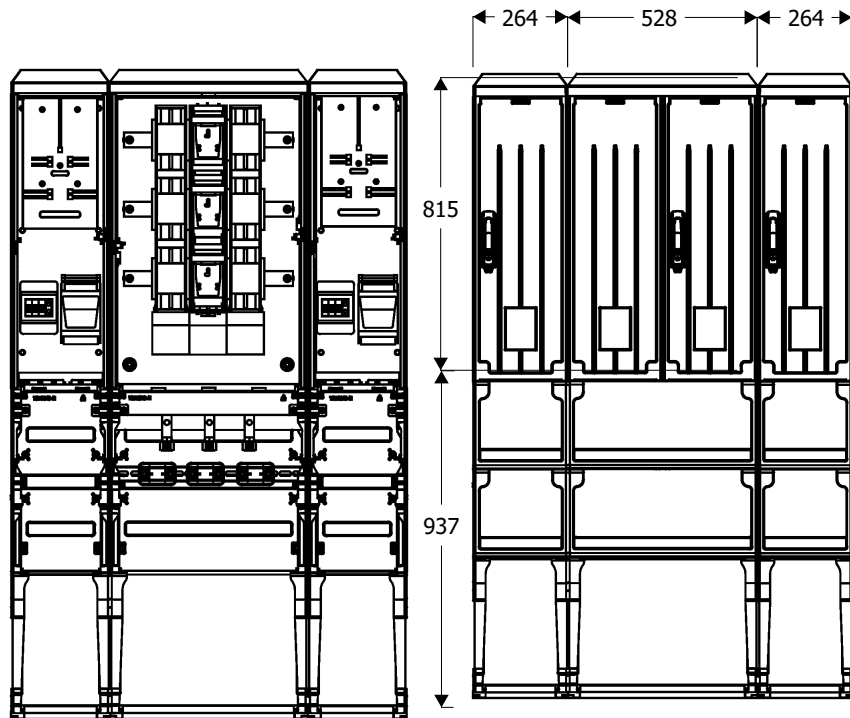
Widok złącza
