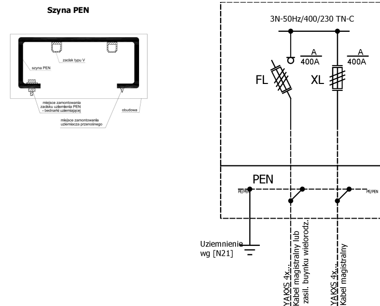
Schemat elektryczny
