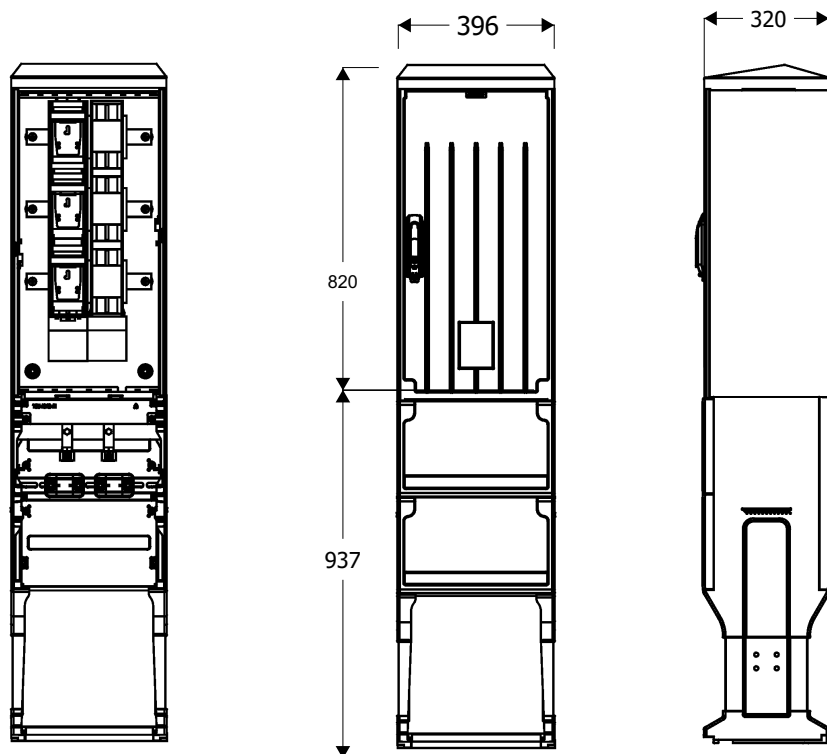
Widok złącza
