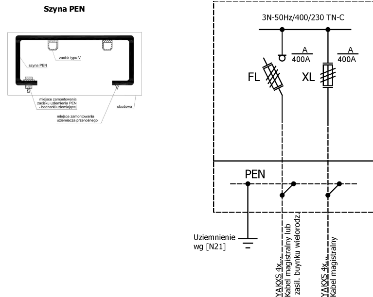
Schemat elektryczny
