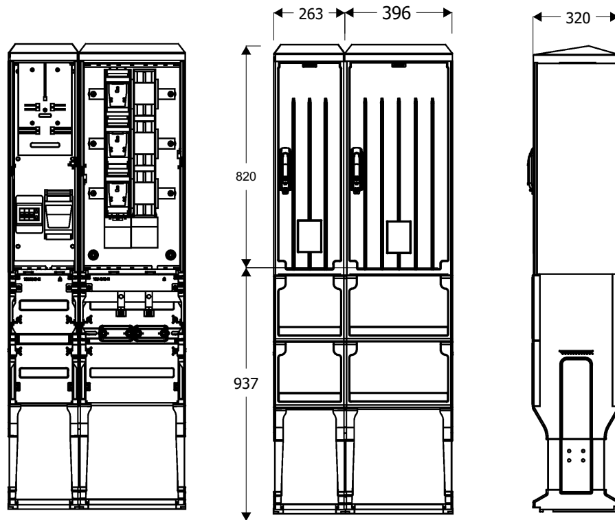
Widok złącza
