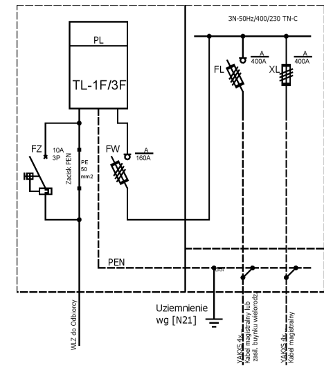
Schemat elektryczny
