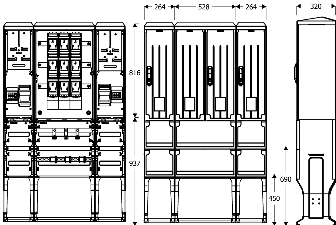
Widok złącza
