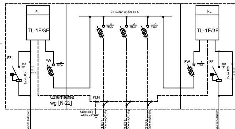
Schemat elektryczny
