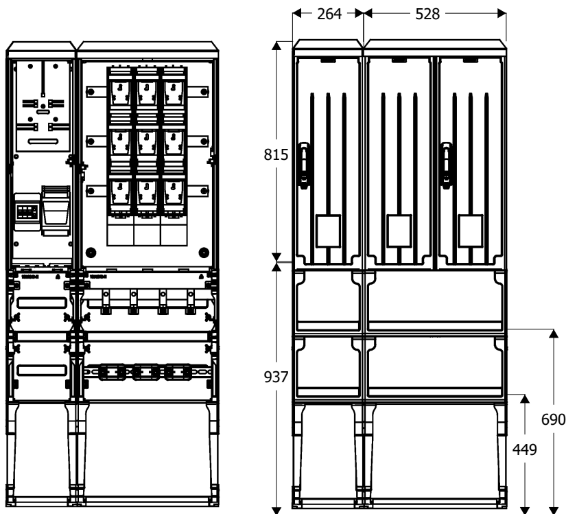
Widok złącza
