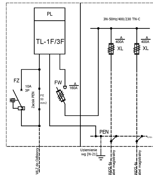
Schemat elektryczny
