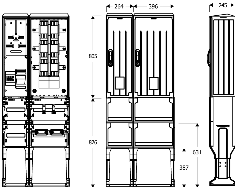
Widok złącza
