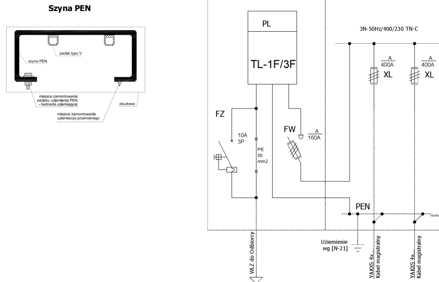
Schemat elektryczny
