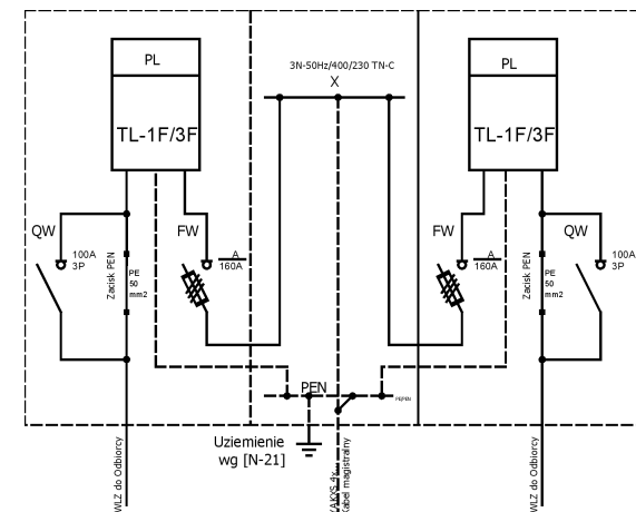
Schemat elektryczny
