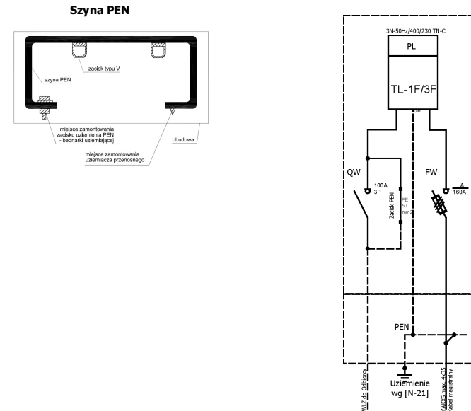
Schemat elektryczny
