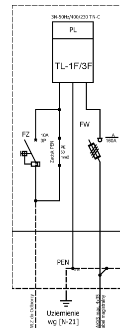
Schemat elektryczny
