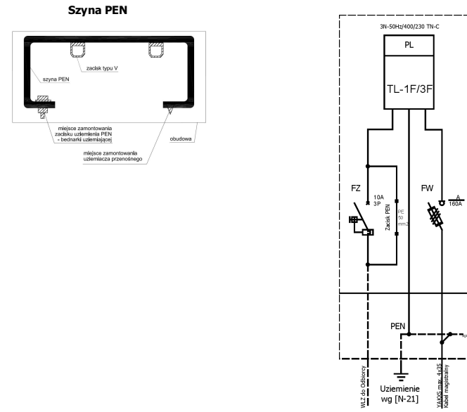
Schemat elektryczny
