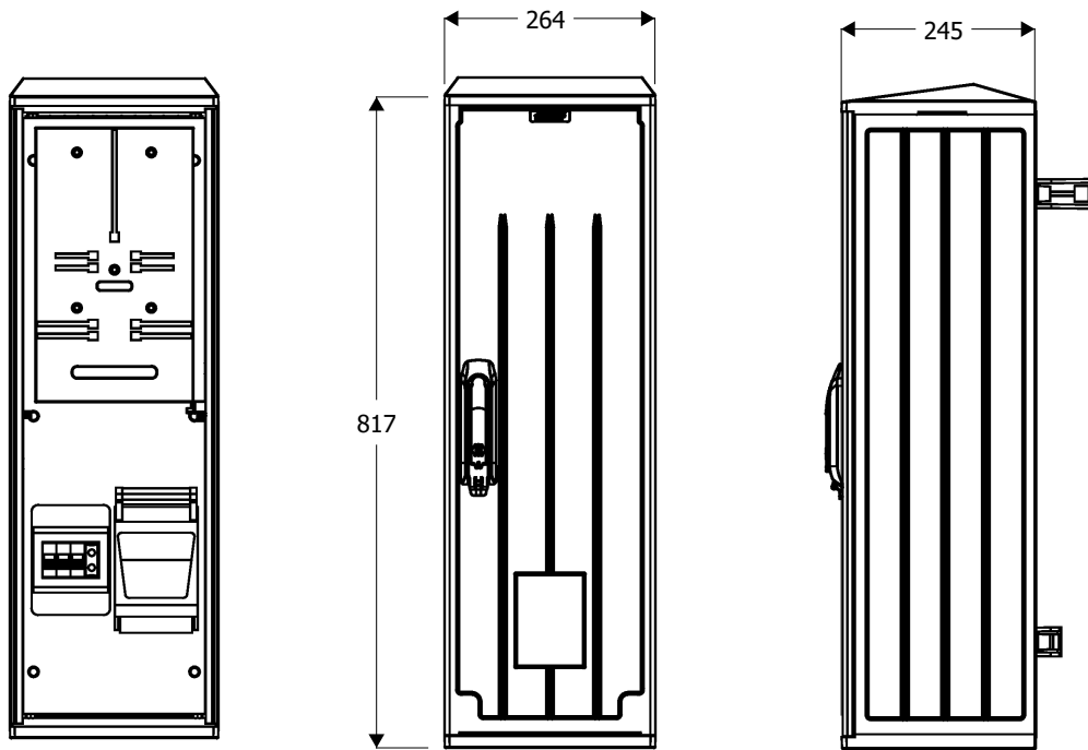
Widok złącza
