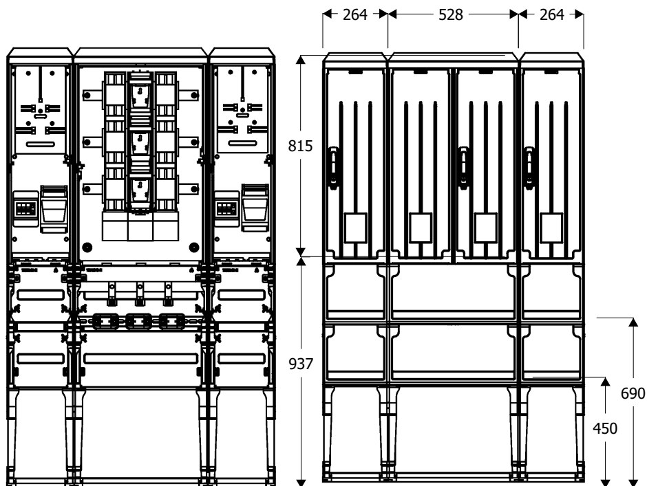
Widok złącza
