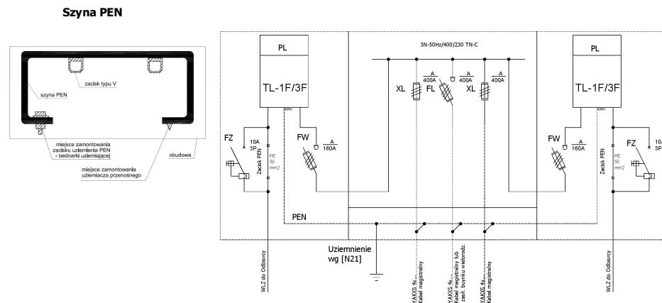
Schemat elektryczny
