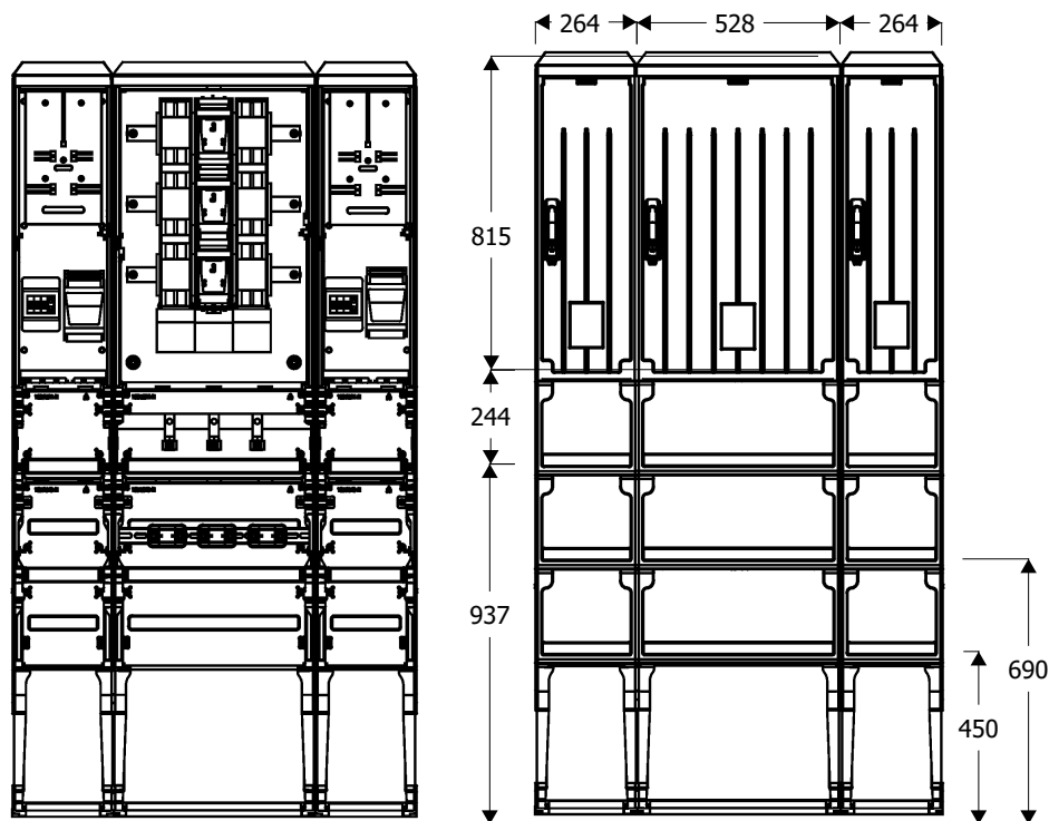
Widok złącza
