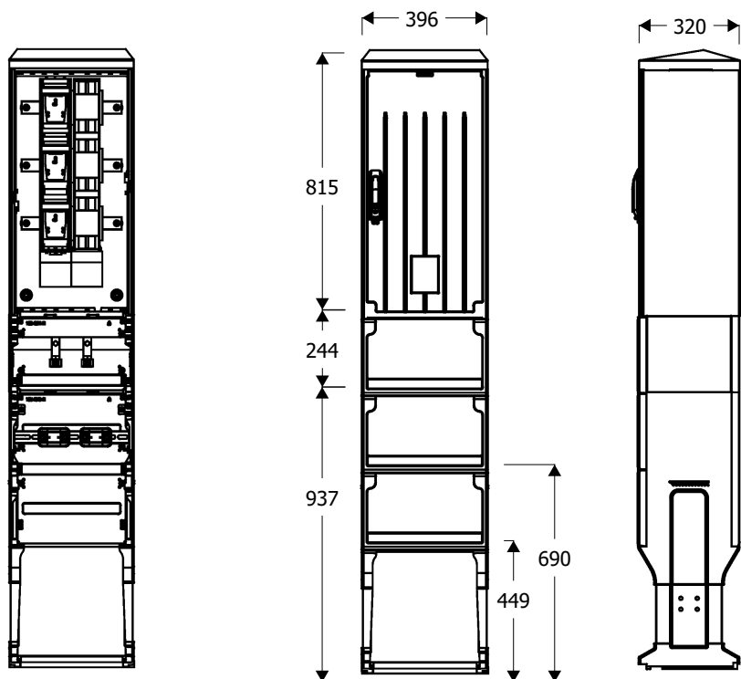
Widok złącza
