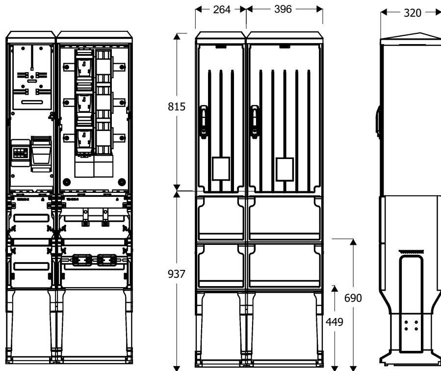
Widok złącza
