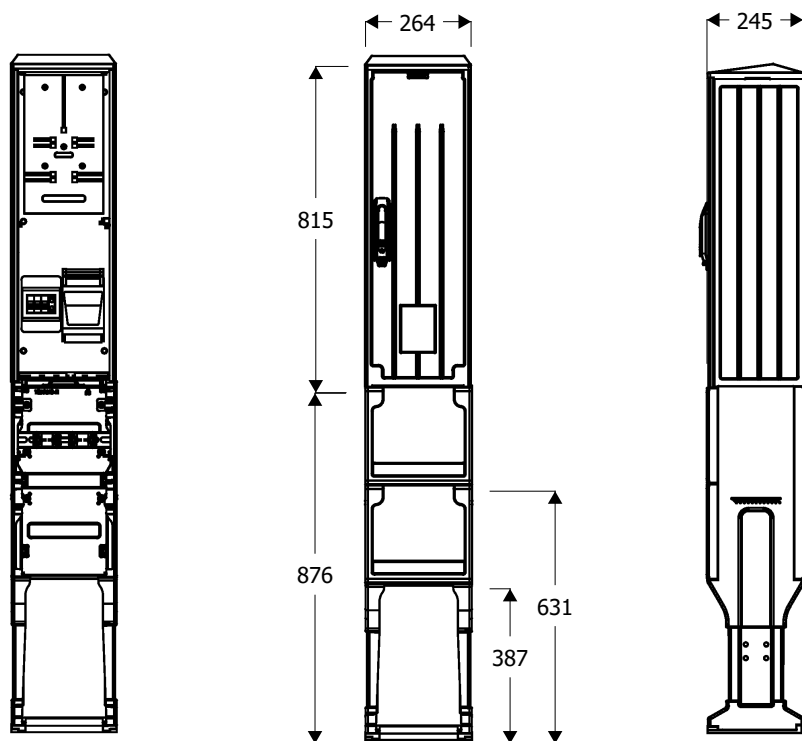
Widok złącza
