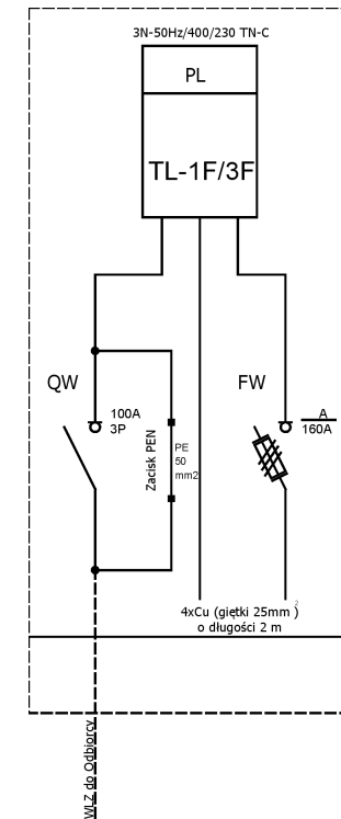
Schemat elektryczny
