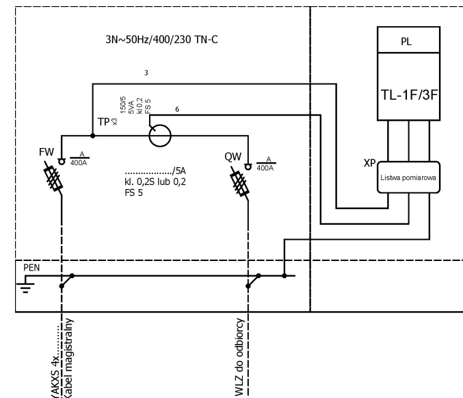
Schemat elektryczny
