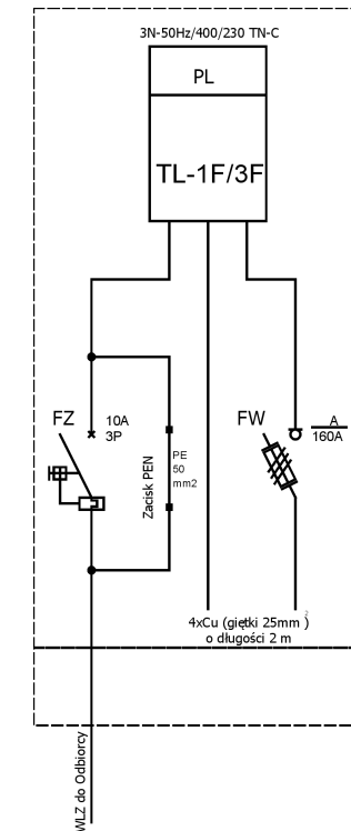
Schemat elektryczny
