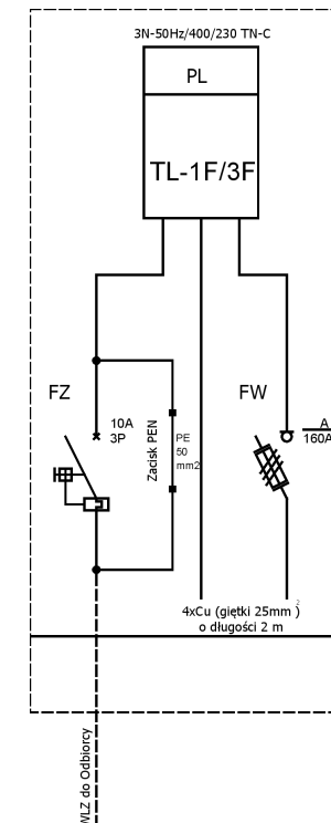
Schemat elektryczny
