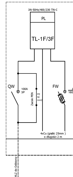
Schemat elektryczny
