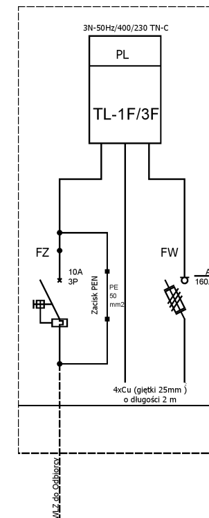
Schemat elektryczny
