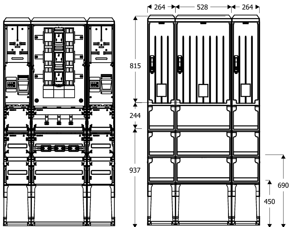
Widok złącza
