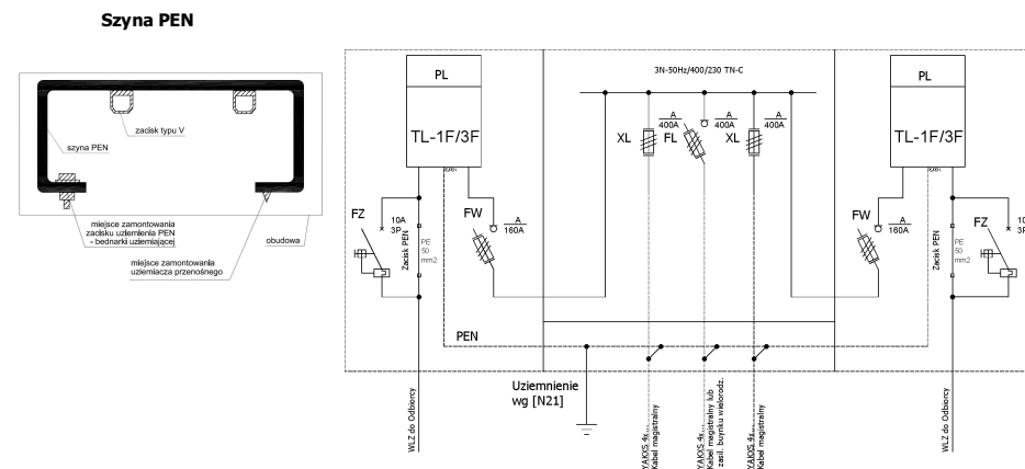
Schemat elektryczny
