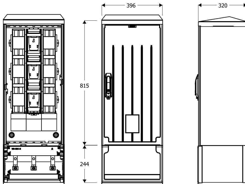
Widok złącza
