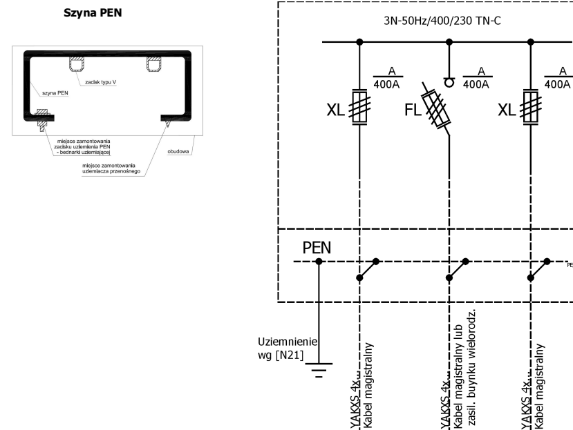
Schemat elektryczny
