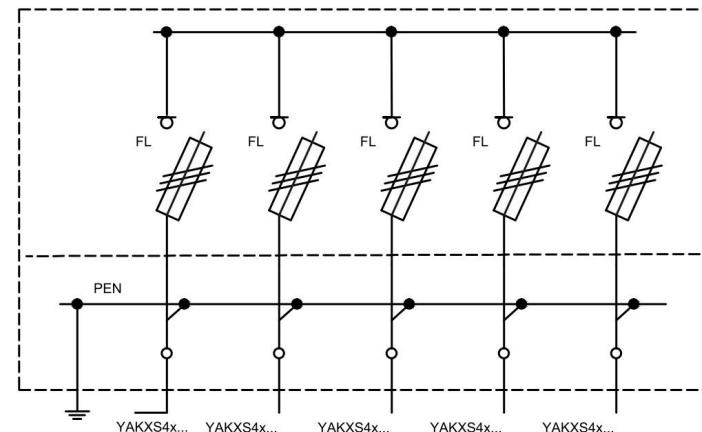
Schemat elektryczny
